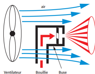
principe et appareil de pulvérisation à pression et jet porté
