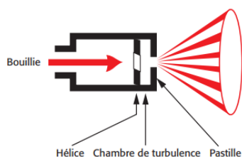
Principe et appareil de pulvérisation à pression et jet projeté
